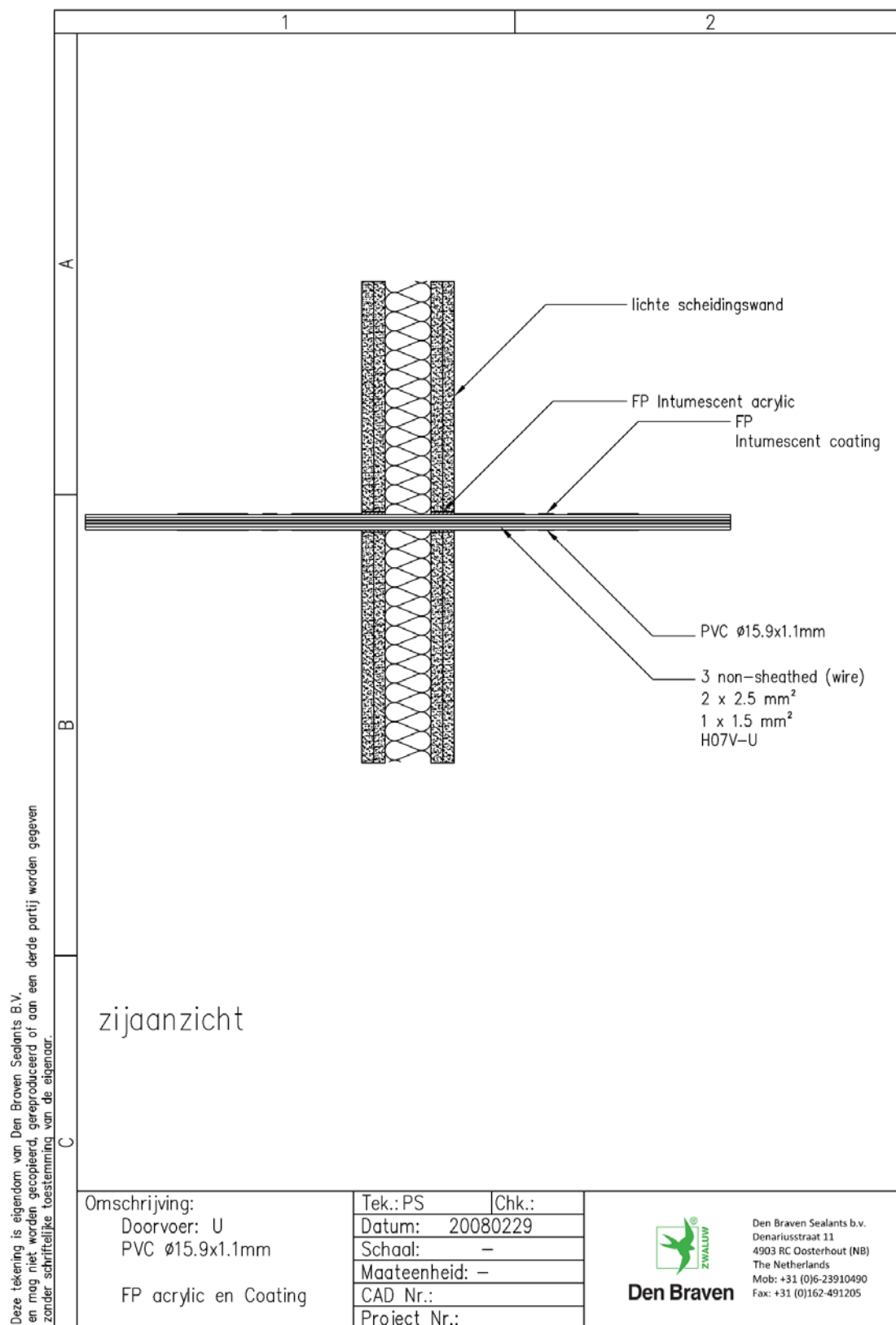
Figuur 34. Detail proefstuk U, gebaseerd op 2008-Efectis-R0458[Rev.2]
