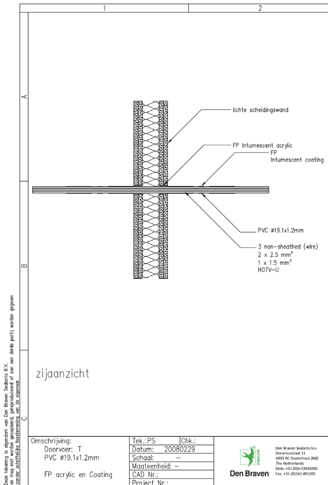
Figuur 33. Detail proefstuk T, gebaseerd op 2008-Efectis-R0458[Rev.2]
