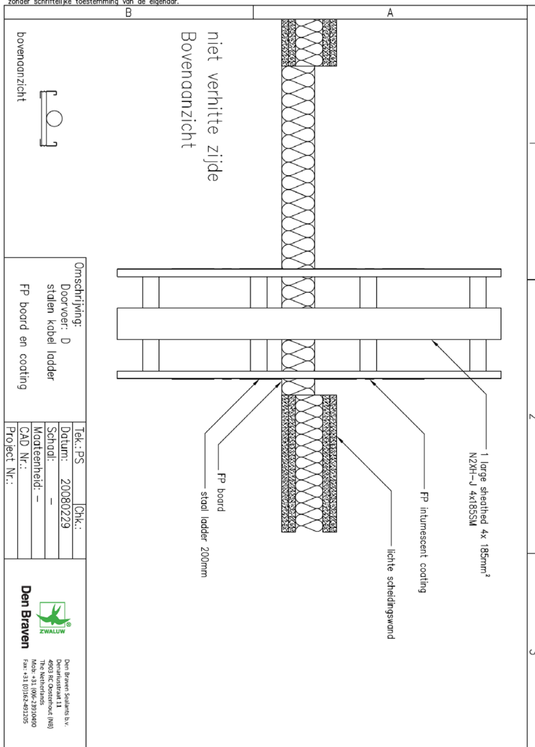
Figuur 24. Detail proefstuk D d.d. 06-06-2008, gebaseerd op 2008-Efectis-R0451
