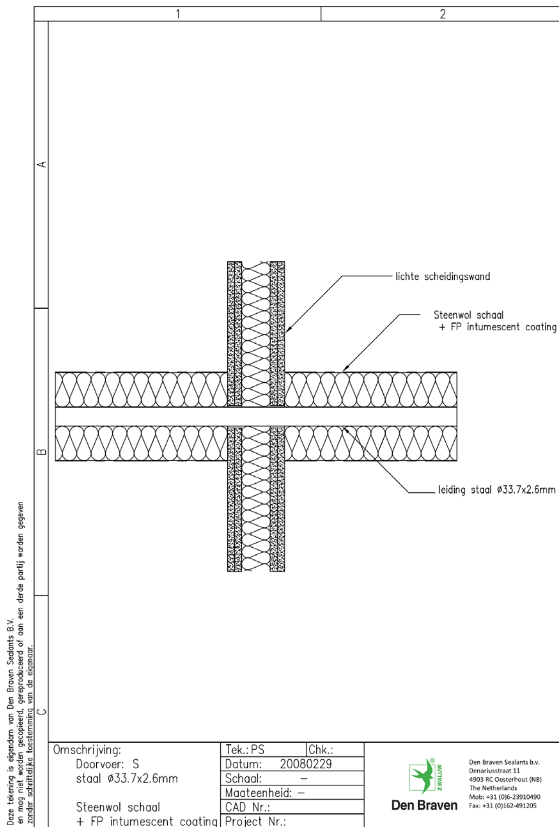
Figuur 31. Detail proefstuk S, gebaseerd op 2008-Efectis-R0456[Rev.1]
