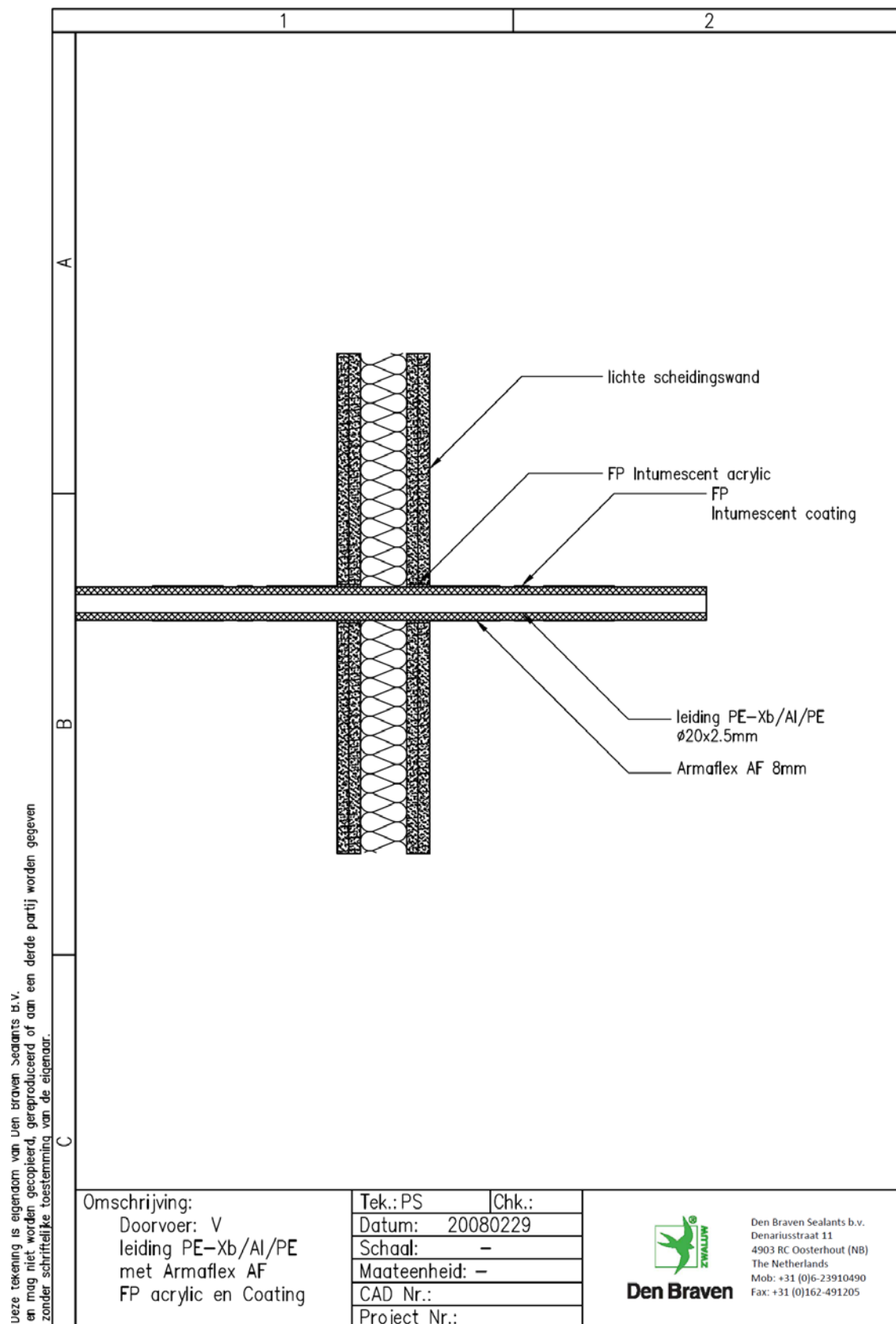
Figuur 37. Detail proefstuk V, gebaseerd op 2008-Efectis-R0461[Rev.1]
